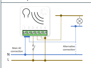
Schéma pour le contrôle d'une charge raccordée au même système d'alimentation standard
