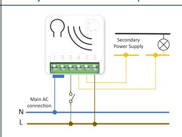
Schéma pour le contrôle d'une charge raccordée à un système d'alimentation indépendant
